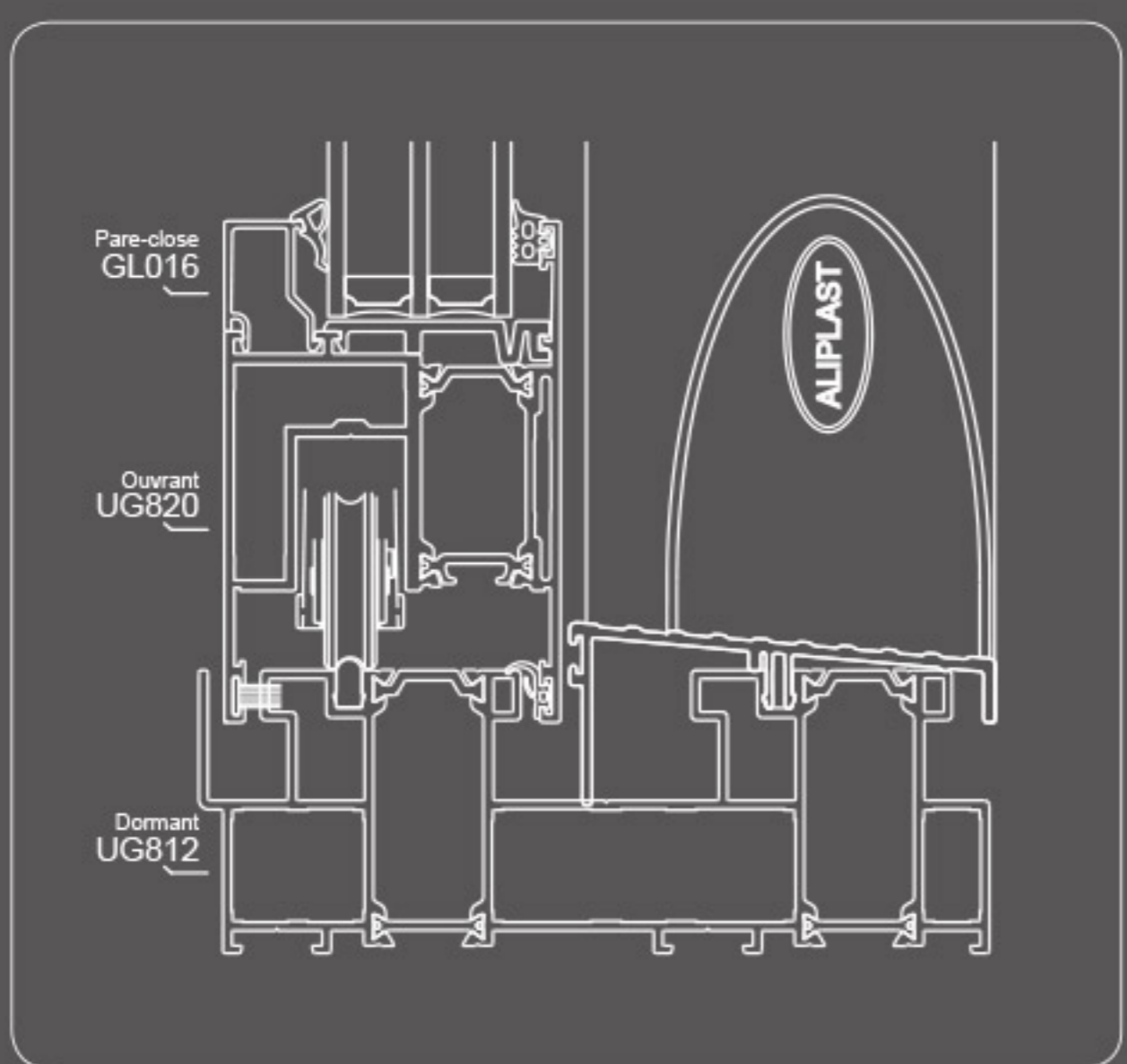
Profils principaux Ultraglide
