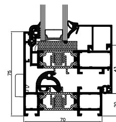
Coupe de fenêtre ouvrante
