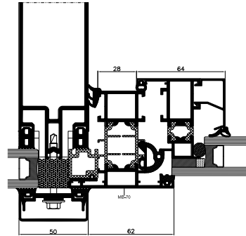
Coupe de fenêtre ouvrante en façade rideau
