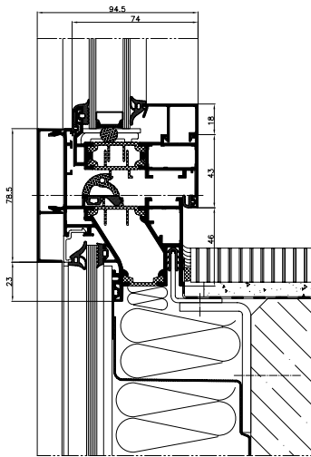
Coupe de fenêtre ouvrante
