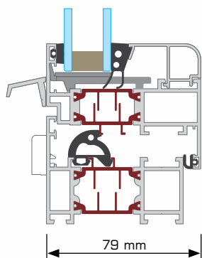
Coupe de fenêtre ouvrante
