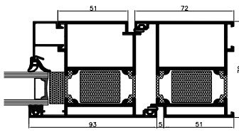
Coupe de porte
