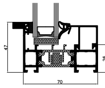
Coupe de fenêtre fixe
