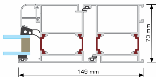
Coupe de porte
