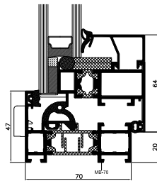
Coupe de fenêtre ouvrante
