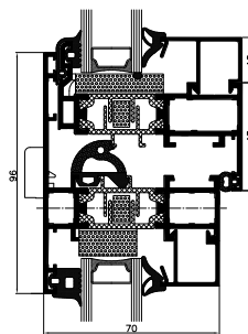
Coupe de fenêtre ouvrante et fenêtre fixe
